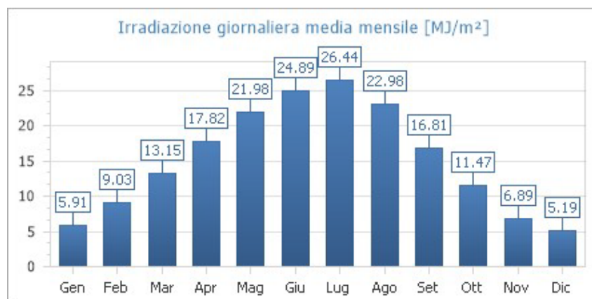
Fig. 1: Irradiazione giornaliera media mensile sul piano orizzontale [MJ/m 2 ]- Fonte dati: UNI 10349 - Località di riferimento: BENEVENTO (BN)/CAMPOBASSO (CB)
