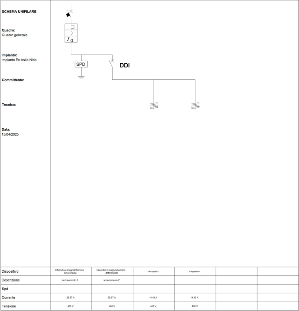
Fig. 5: Schema unifilare quadro "Quadro generale"
