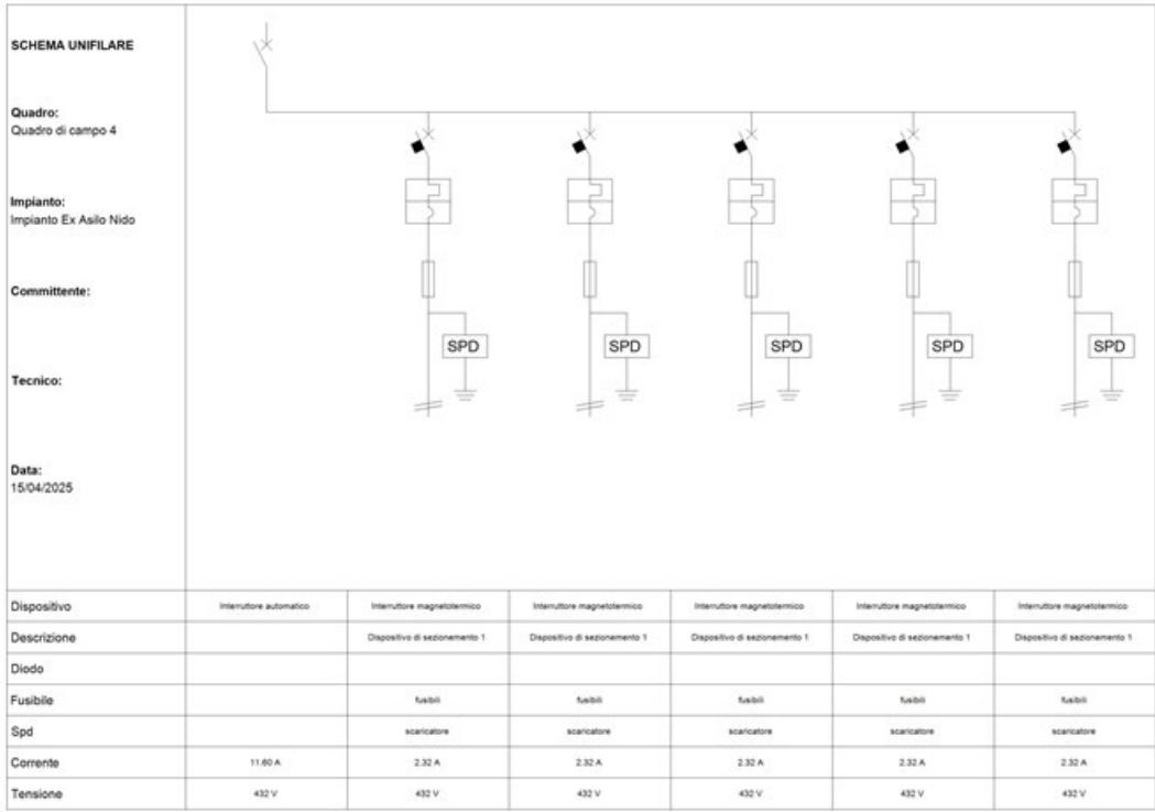
Fig. 9: Schema unifilare quadro "Quadro di campo 4"
