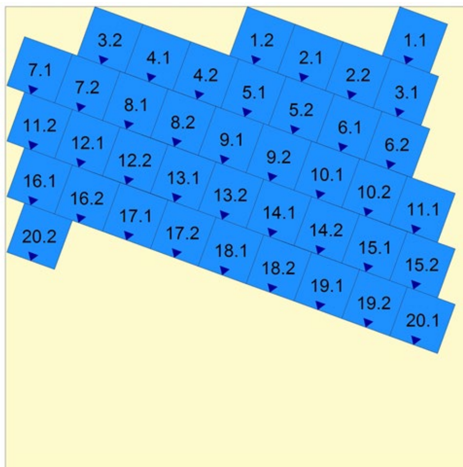
Fig. 4: Posizionamento dei moduli del generatore Generatore1
